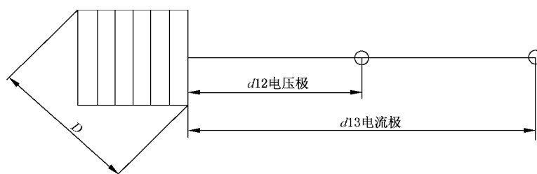
图 C.2 直线形布置
